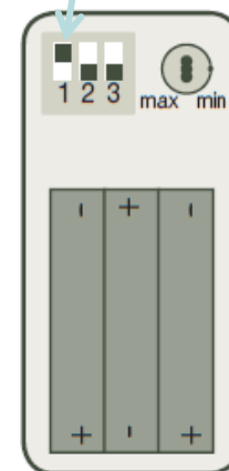
Sensor PIR trådløs type 44-045
